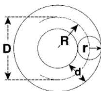
Torus
